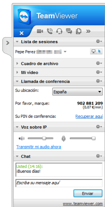
El Panel de TeamViewer de control remoto.
